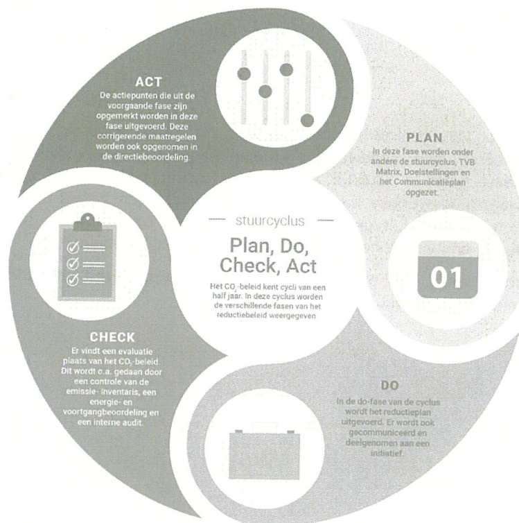
Figuur 1: PDCA-cyclus
